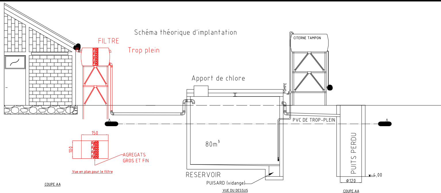
COUPE AA
